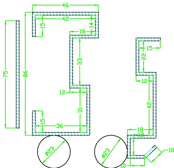
LAMIERA PRESSOPIEGATA 20/10
